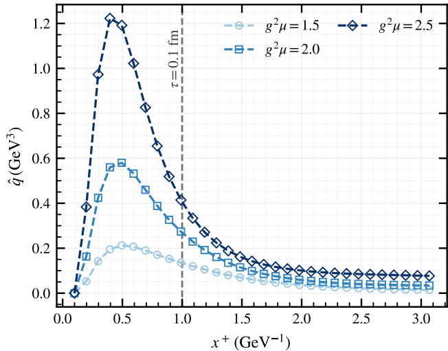
(a) Jet quenching parameter
